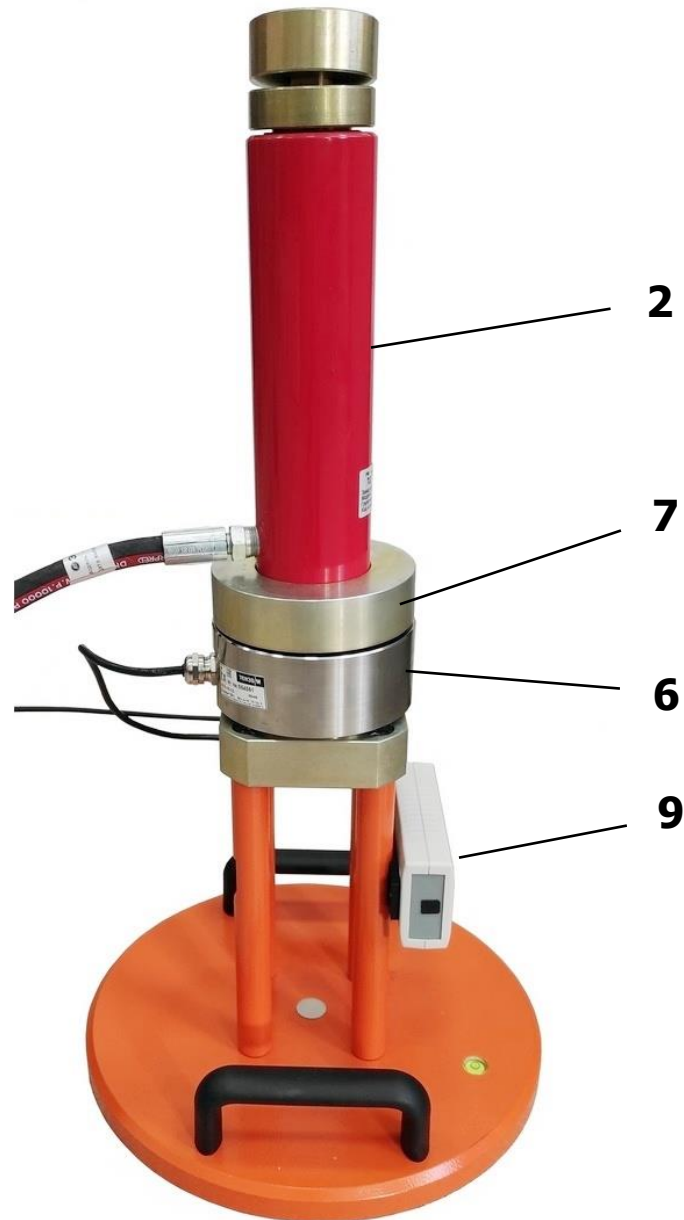
Рисунок 5 – Нагрузочная плита 300 мм с установленным гидроцилиндром
